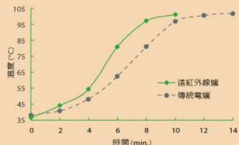
烘焙過程蛋糕中心溫度之變化
